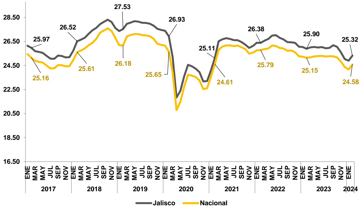
Figura 27. Precio promedio mensual de la gasolina premium Jalisco y México, enero 2017 a febrero 2024, a pesos constantes
