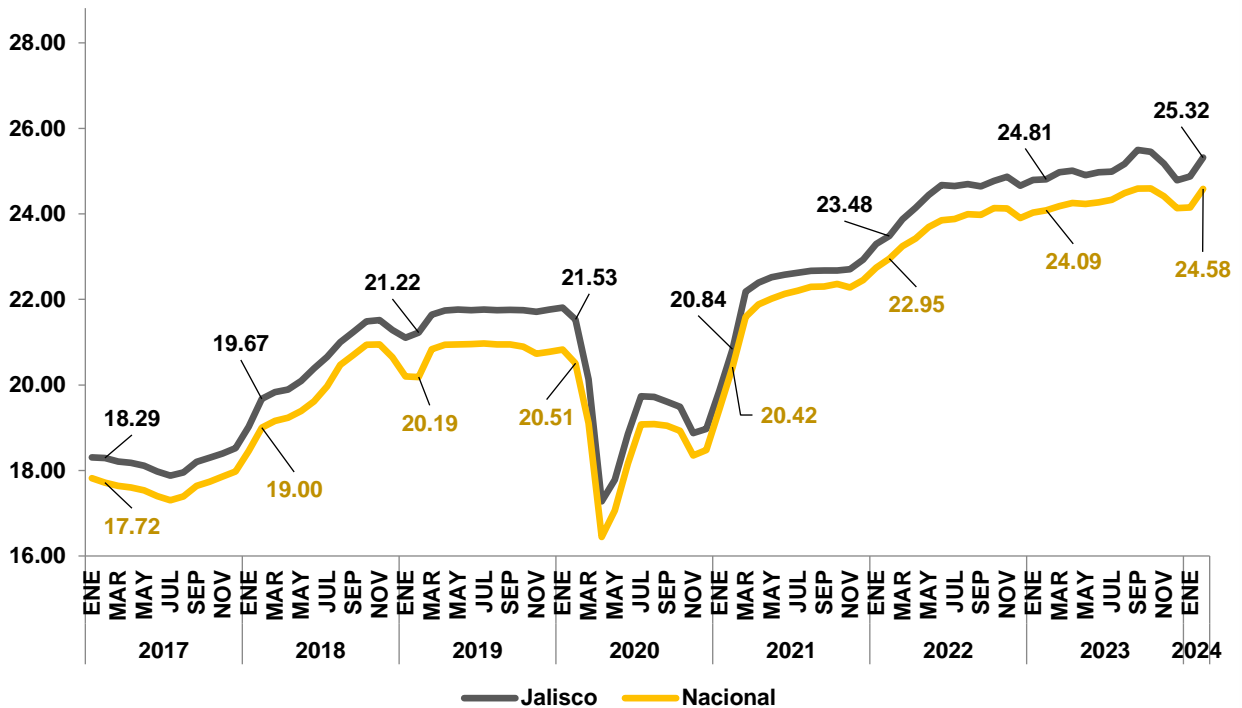
Figura 28. Precio promedio mensual de la gasolina premium Jalisco y México, enero 2017 a febrero 2024, a pesos corrientes
