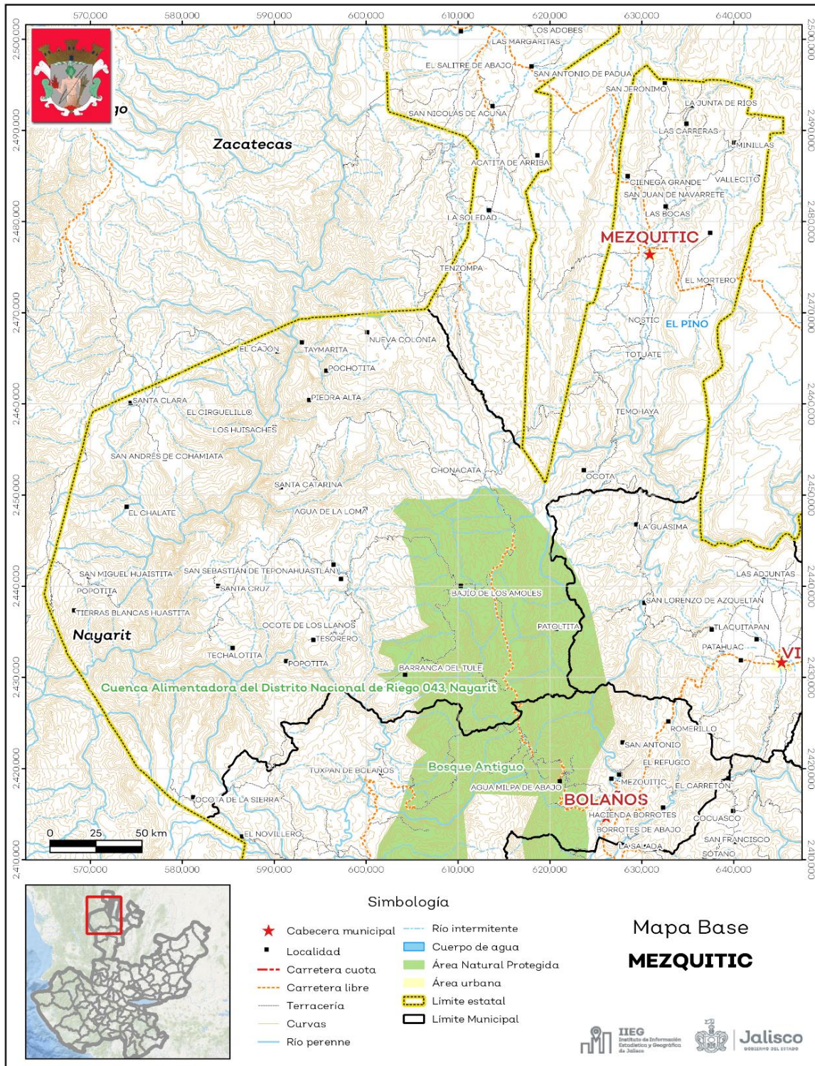
Mapa 1. Base
