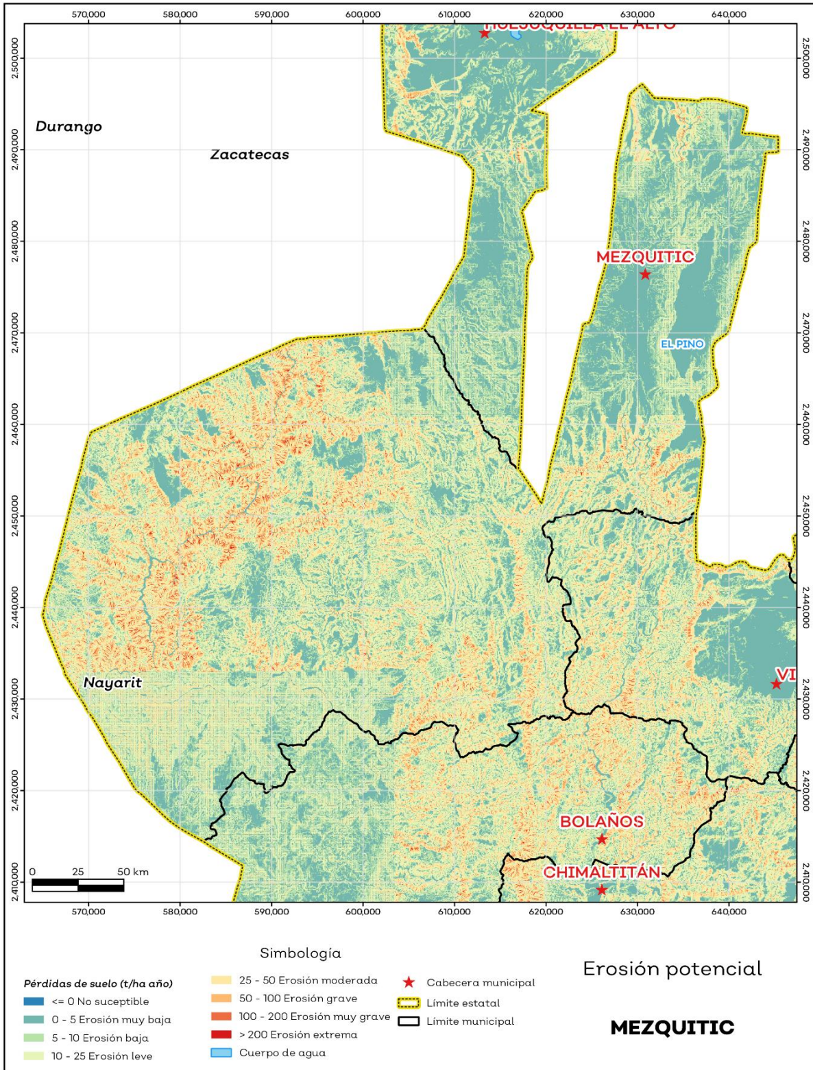
Mapa 8. Erosión potencial
