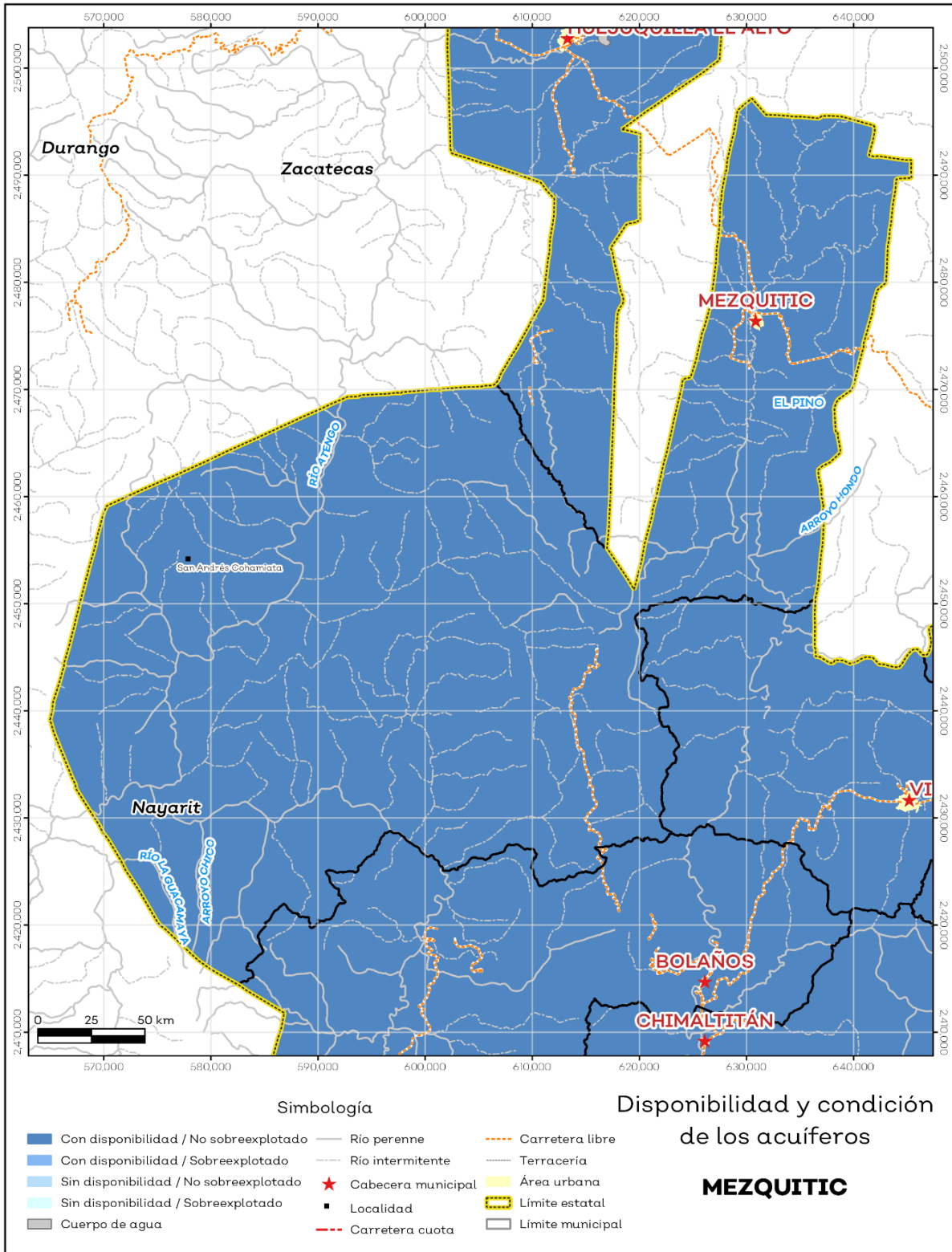
Mapa 6. Acuíferos
