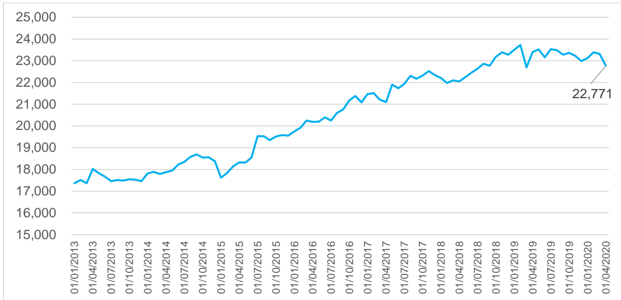
Figura 14. Personal ocupado total en la industria del plástico y hule, enero 2013 – abril 2020
